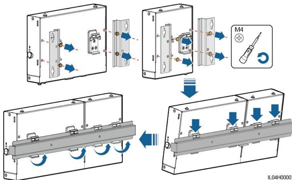
3-6. ábra Telepítés vezetősínre
