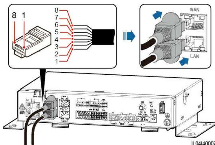
4-10. ábra Ethernet-kábel csatlakoztatása
