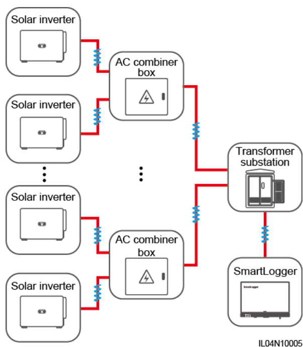
4-4. ábra MBUS-hálózat
