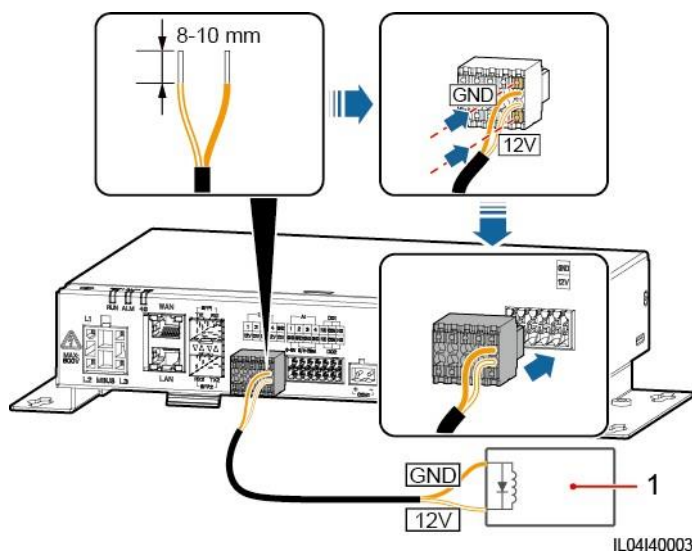
4-7. ábra A kimeneti erősáramú kábel bekötése
