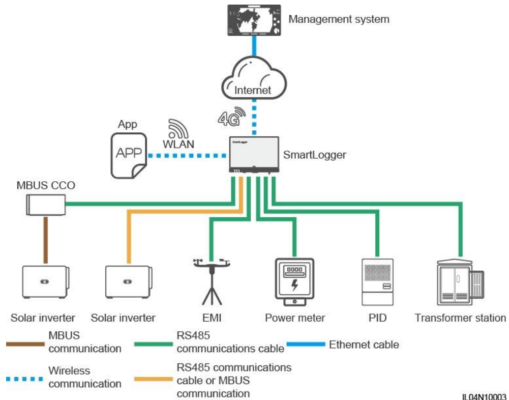
2-5. ábra 4G-hálózat
