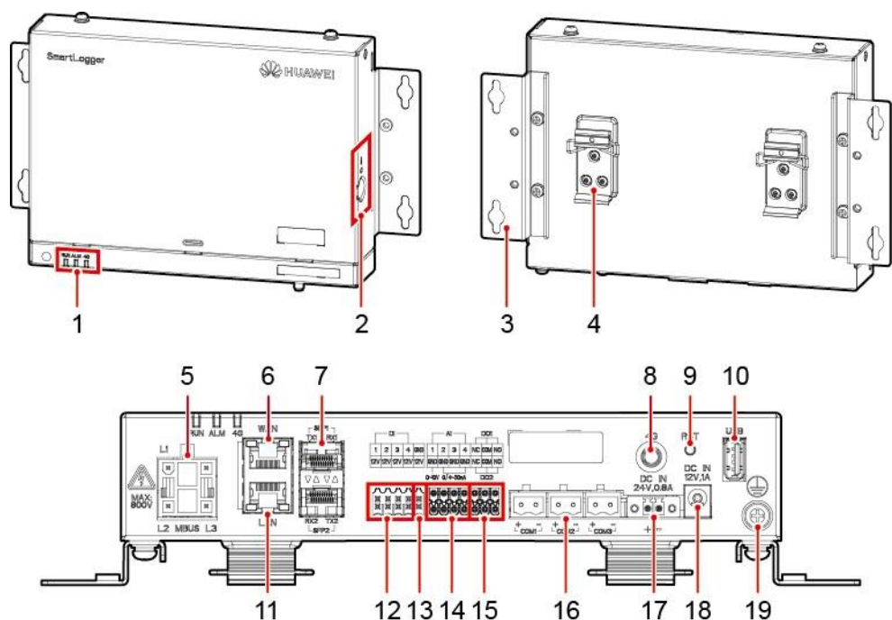
2-7. ábra SmartLogger
