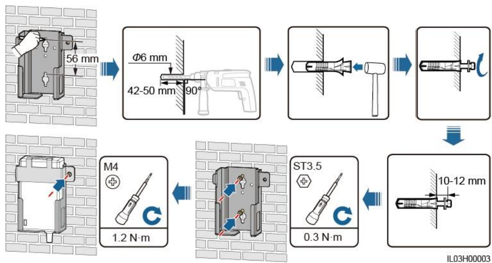
3-9. ábra Fali telepítés (1. mód)
