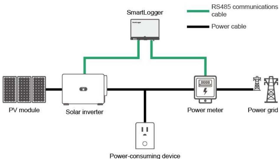
6-44. ábra Hálózati ábra (megszakító nélkül)
