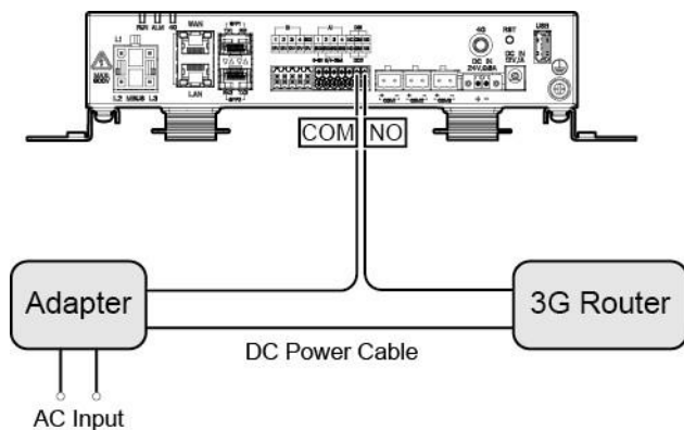
8-5. ábra Csatlakoztatás a DO-portba
