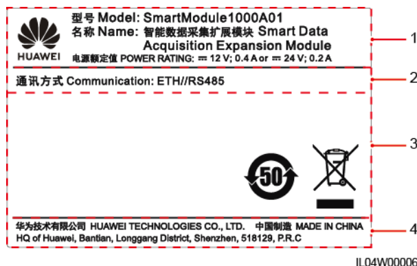
2-10. ábra Típustábla
